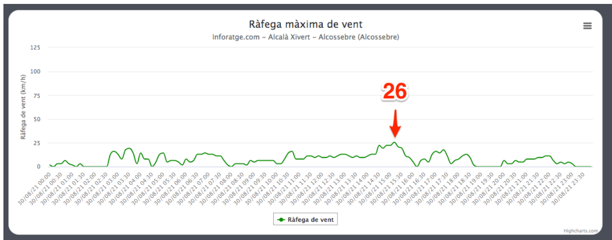
Ráfegas de viento registradas en ALCOSSEBRE el 30/08/21 (en km/h)
