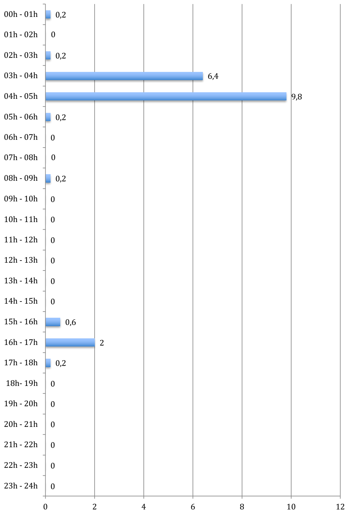
Cantidades de lluvia registradas por horas en ALCALÀ DE XIVERT el 30/08/21 (en l/m²)
