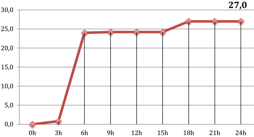
Evolución lluvia acumulada en ALCOSSEBRE el 30/08/21 en períodos de 3 horas (en l/m 2 )
