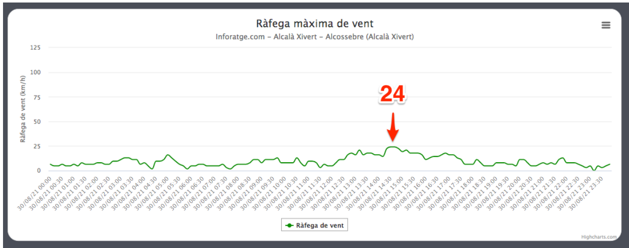
Ráfegas de viento registradas en ALCALÀ DE XIVERT el 30/08/21 (en km/h)
