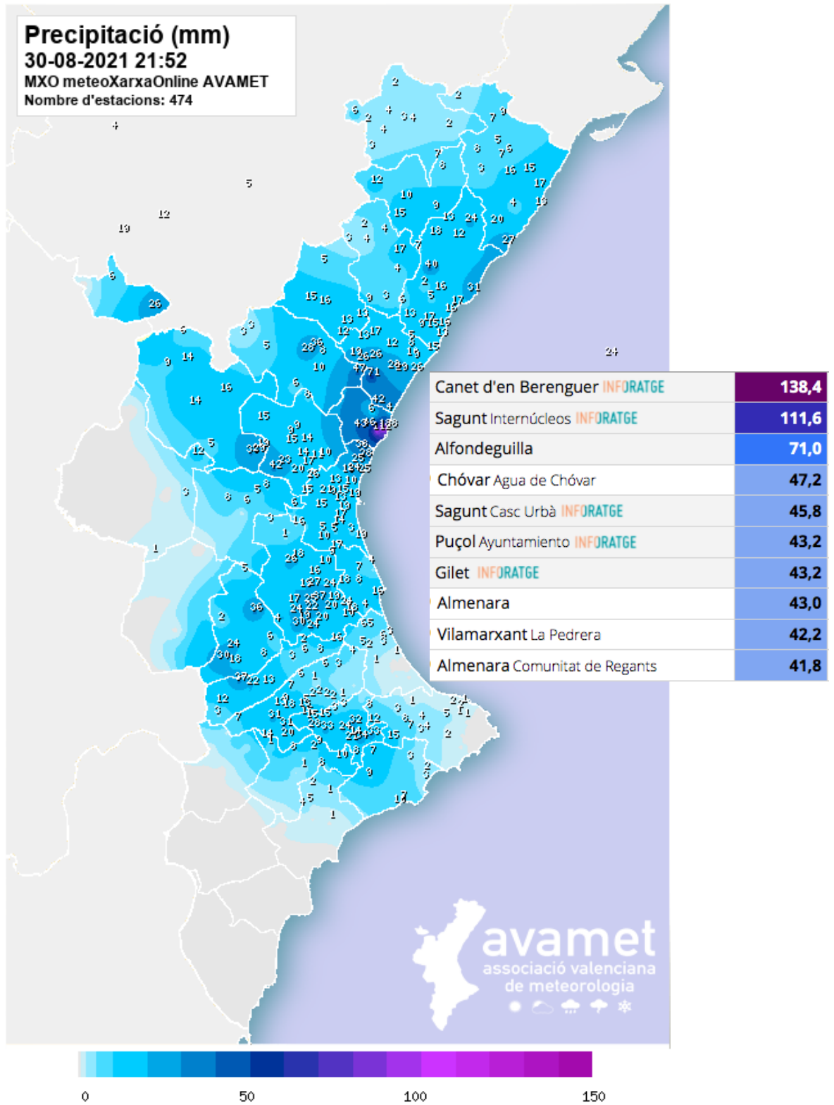
Distribución y precipitaciones máximas registradas el lunes 30-08-2021 (Fuente: AVAMET- Inforatge)
