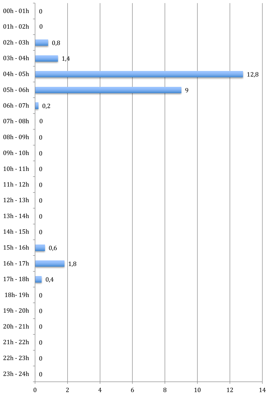
Cantidades de lluvia registradas por horas en ALCOSSEBRE el 30/08/21 (en l/m²)
